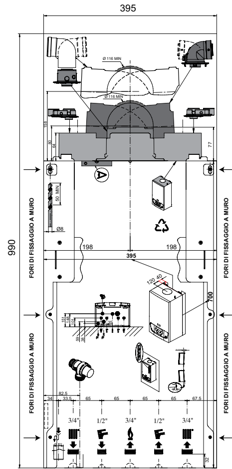
Dima di installazione telaio distanziale 40 mm (4 viti di fissaggio incluse)
